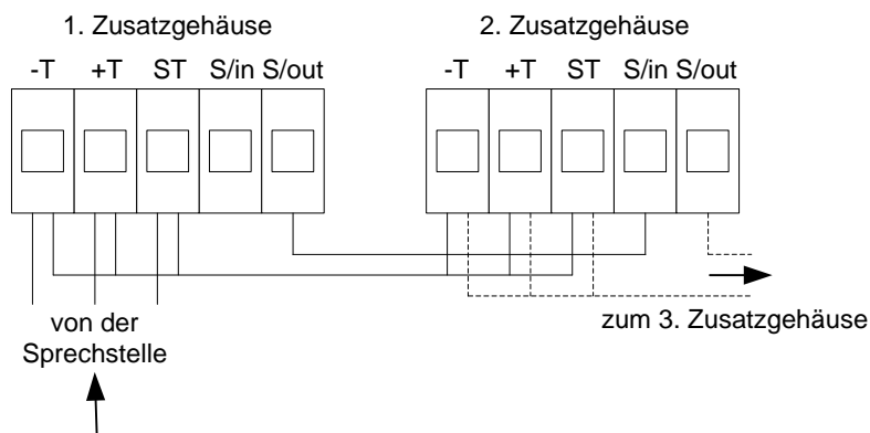
Anschlussschema für das Zusatztastenfeld AWC-06
