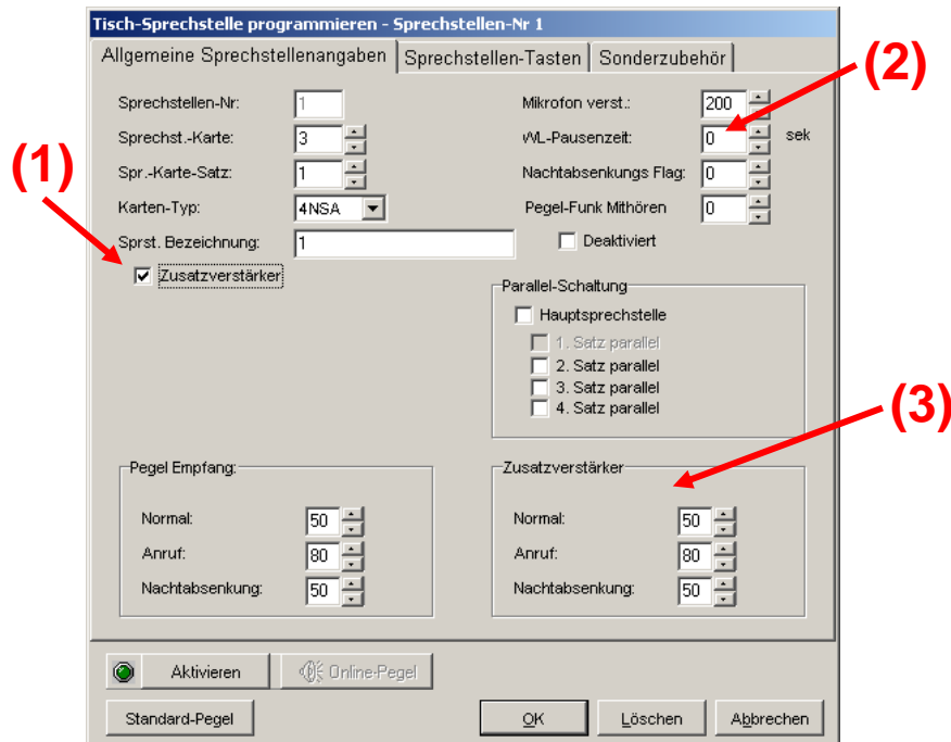
Abb. 3: ICS-Konfigurationsmaske für Tischsprechstellen
