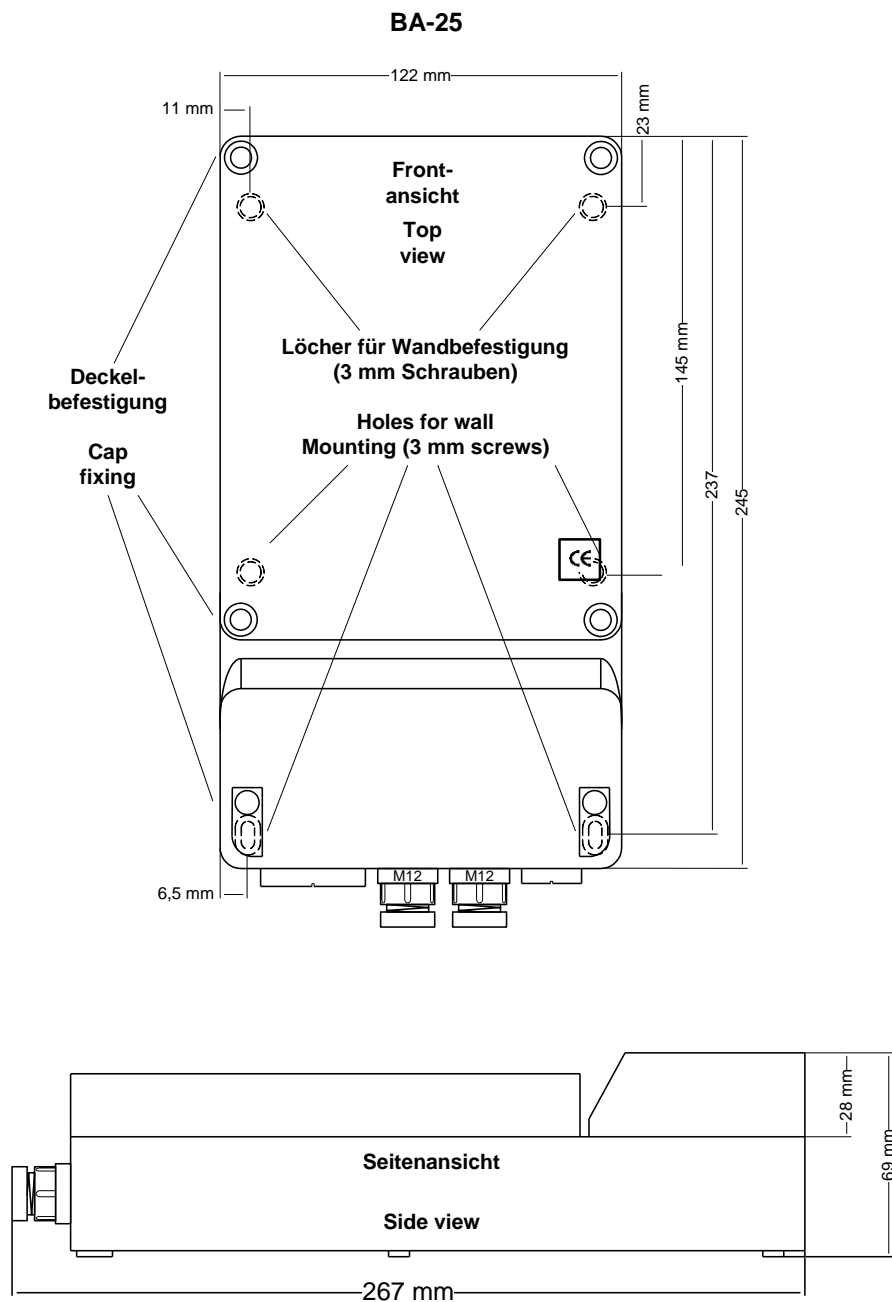
Abb. 2: Maßzeichnung BA-25
